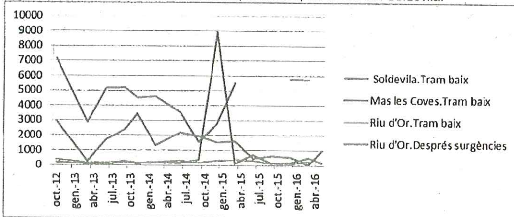
Evolució del contingut en clorurs (mg/L) en tributaris del riu Llobregat( pic corresponent al trencament del col·lector)
