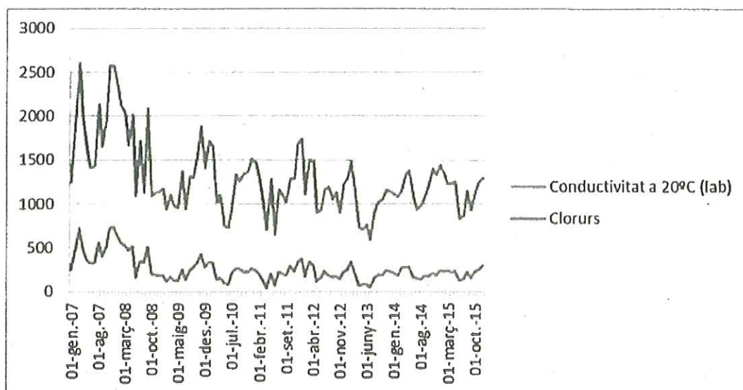
Evolució de clorurs (mg/L) i conductivitat elèctrica (µS/cm) en el riu Llobregat, en l'estació ubicada aigües avall de Sallent, després de l'activitat minera.
